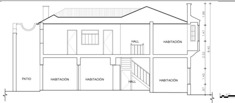
Corte longitudinal
